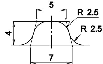
DETTAGLIO DELLA TACCA A90° RISPETTO A.A.S. SCALA 3:1
